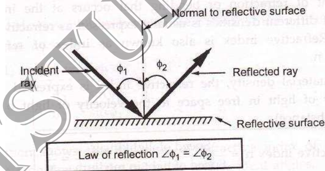
Fig. 1.6.2 Reflection
