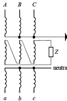
(d) Neutral point transformer with compensation delta
